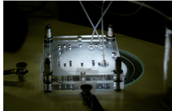
foto van een experiment met kleine Y reactor (vouwchip) en laminaire flow.
